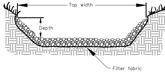
Trapezoidal Riprap Channel
