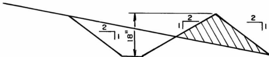
DIVERSION DITCH
